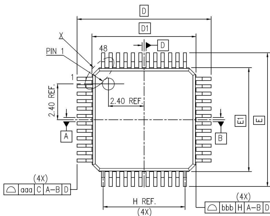
图 23 LQFP48 封装图
