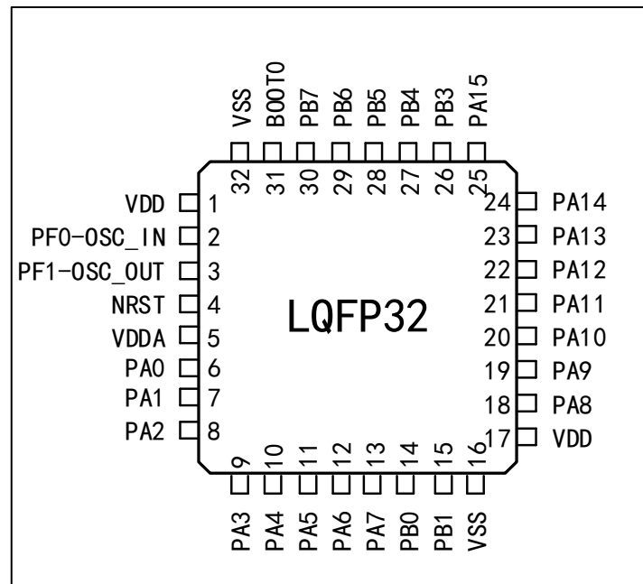
图 3 APM32E030x8 系列 LQFP32 引脚分布图
