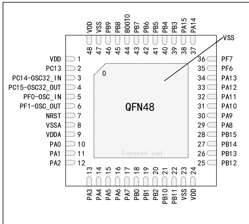
图 4 APM32E030x8 系列 QFN48 引脚分布图
