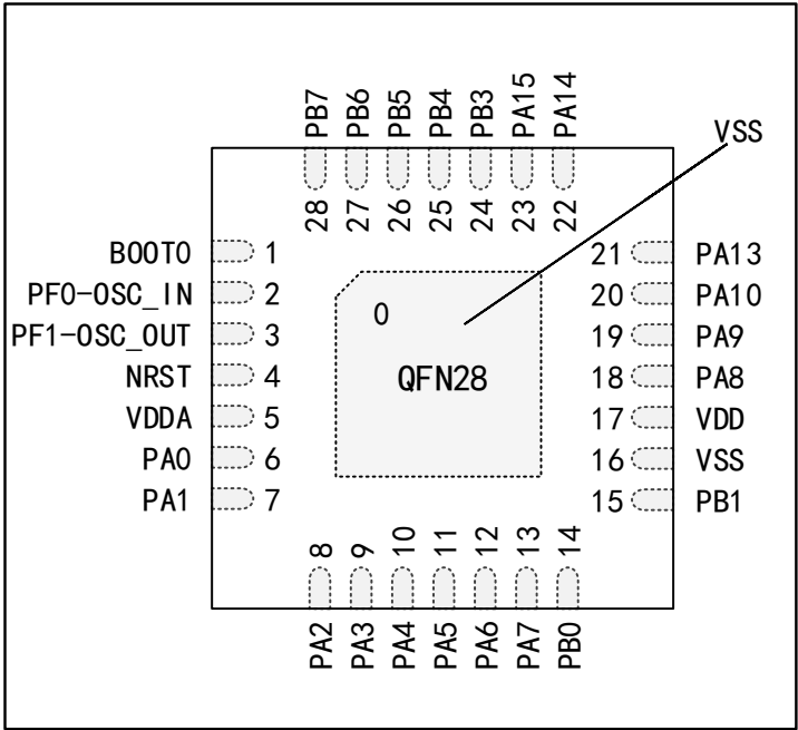
图 6 APM32E030x8 系列 QFN28 引脚分布图
