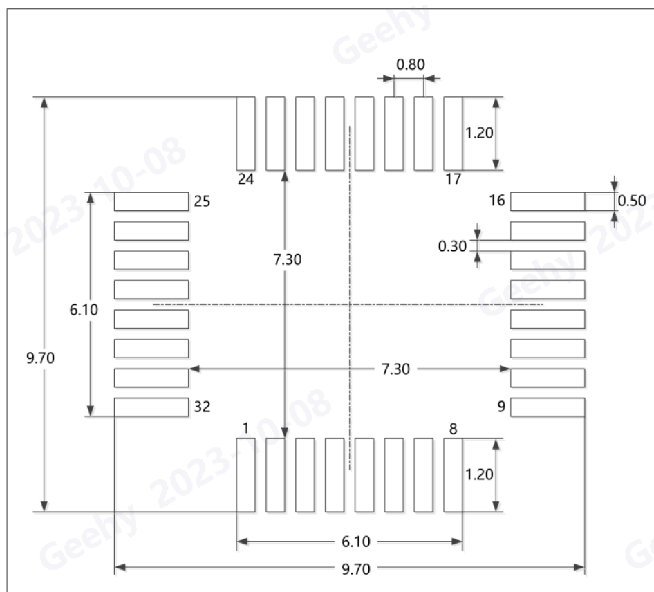
图 30 LQFP32 焊接 Layout 建议
