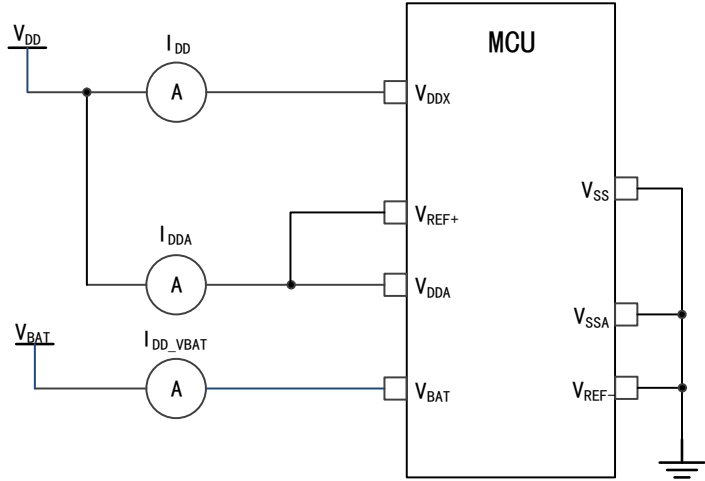
图 14 功耗测量方案
