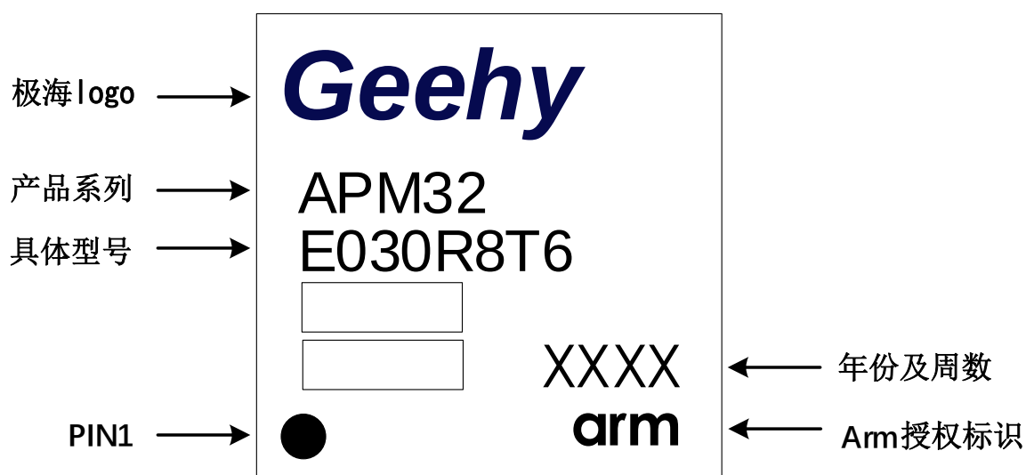
图 22 LQFP64 - 64 引脚, 10 x 10mm 封装标识
