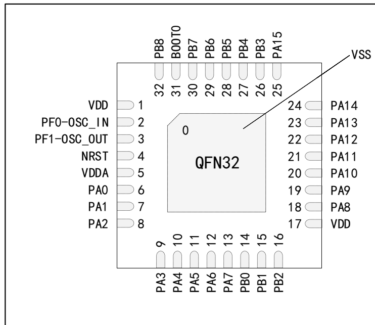
图 5 APM32E030x8 系列 QFN32 引脚分布图
