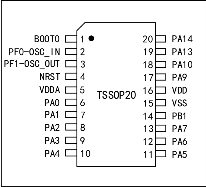
图 7 APM32E030x8 系列 TSSOP20 引脚分布图
