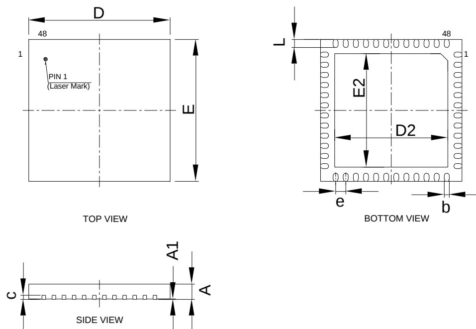
图 26 QFN48 封装图
