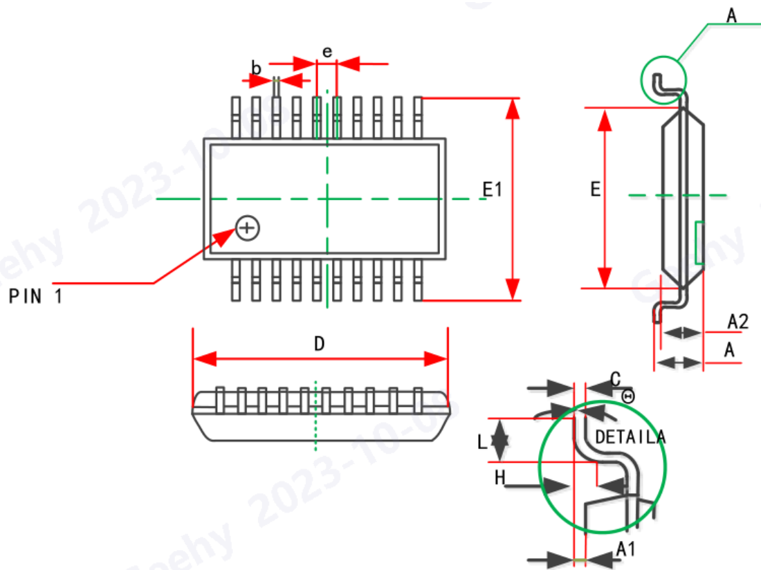
图 38 TSSOP20 封装图
