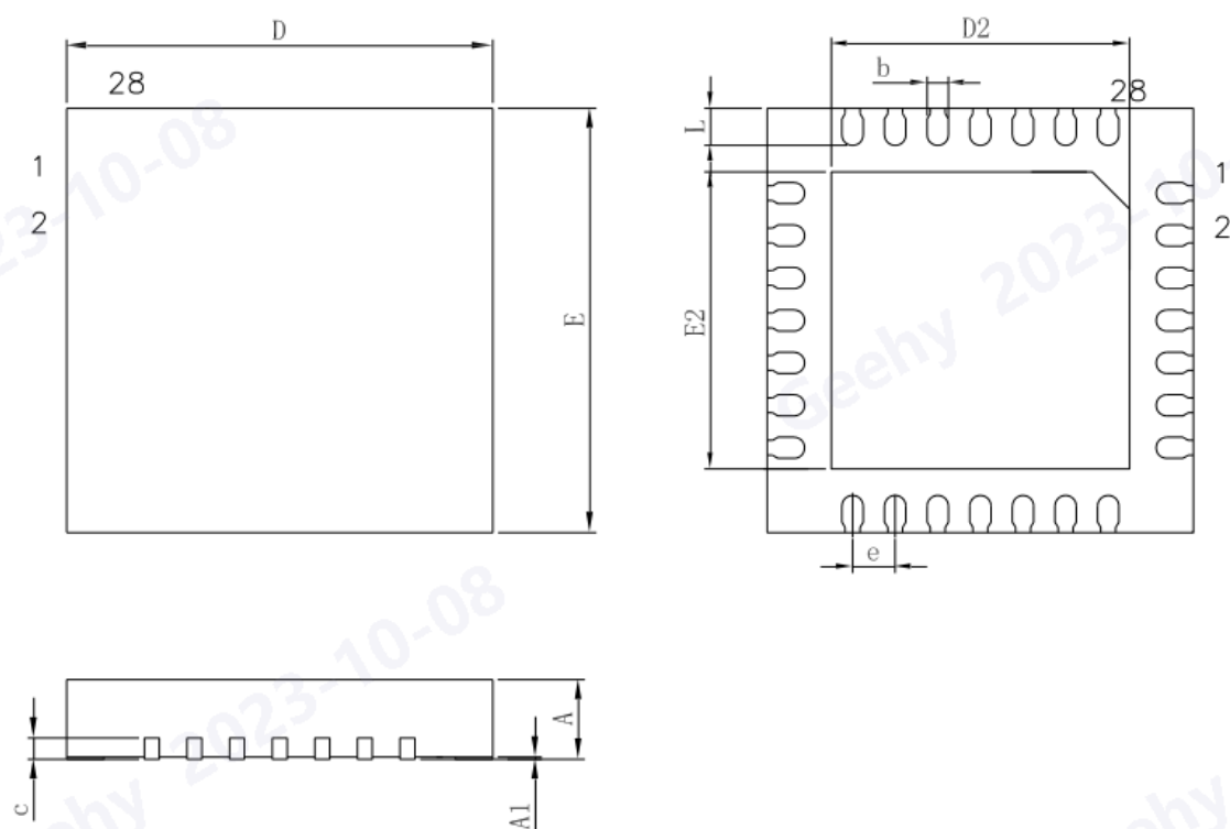
图 35 QFN28 封装图
